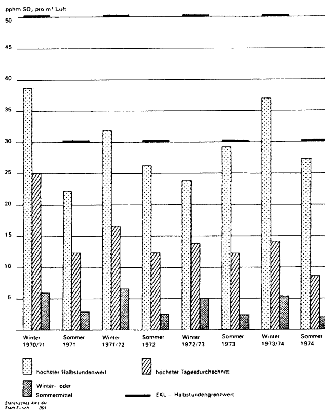
Abbildung 2 Schwefeldioxid-Konzentrationen in der Stadt Zürich. Höchstwerte und Durchschnittswerte der vom Gesundheitsamt der Stadt Zürich seit dem Winter 1970/71 durchgeführten Messungen [20]. 1 pphm = 1 part per hundred million bzw. 0,01 ppm; EKL = Eidg. Kommission für Lufthygiene.
