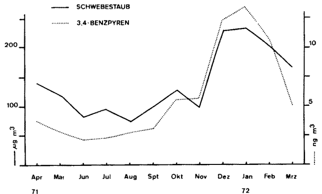
Abbildung 1 Monatsmittelwerte der Schwebestaub- und 3,4-Benzpyrenimmissionen vom April 1971 bis März 1972. Dargestellt sind die Durchschnittswerte der fünf Messstellen in der Stadt Zürich (ohne Uetliberg). Vgl. dazu Tabelle 2 [22].
