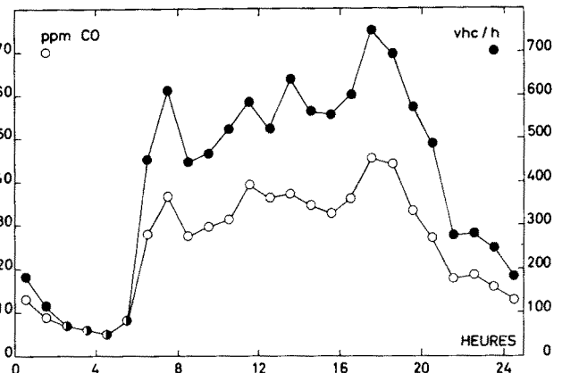
Abbildung 4 Kohlenmonoxid-Konzentration im Strassentunnel von Chauderon bei Lausanne [11]. Stundenmittelwerte im Verlauf eines Tages für das CO (ppm) und für die Anzahl Fahrzeuge pro Stunde (vhc/h).
