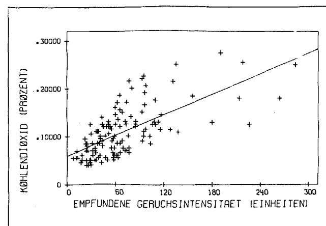
Abb. 2. Zusammenhang zwischen dem Kohlendioxidgehalt (in Prozent) und der empfundenen Geruchsintensität (100 Einheiten entsprechen einem Pyridin-Referenzgeruch von 365 ppb), Korrelationskoeffizient r = 0,67 . Versuch in einer Klimakammer mit unterschiedlichen Belegungen und Luftwechselraten.
